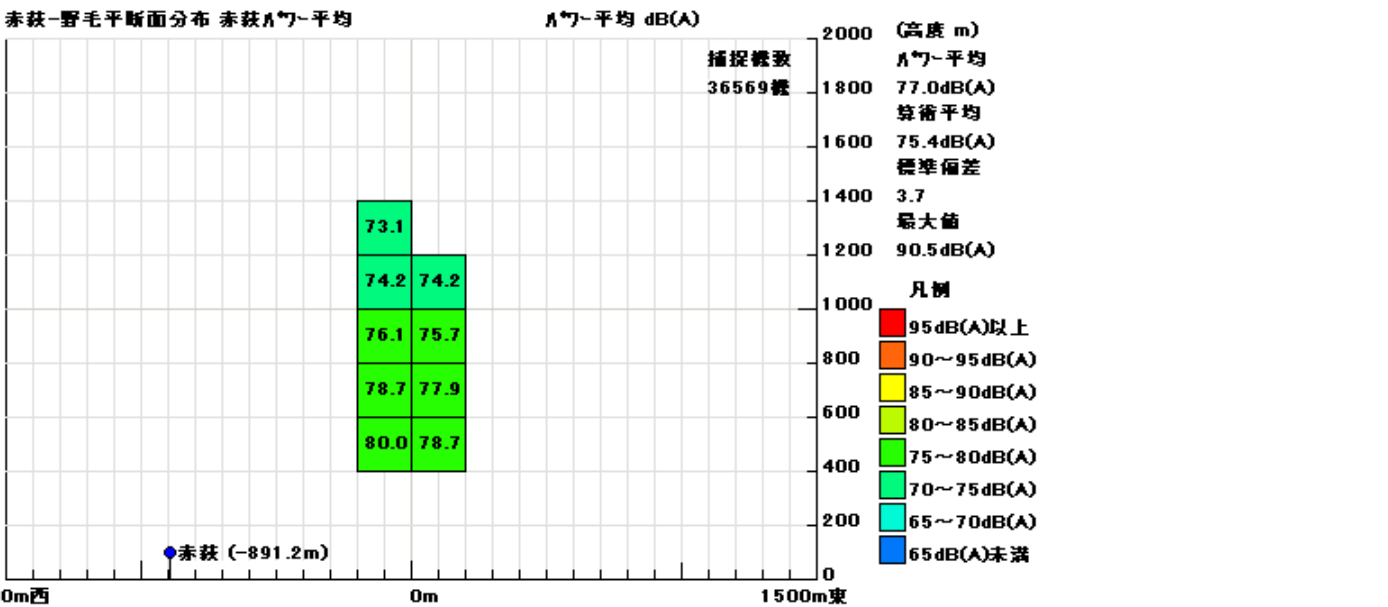
離陸機騒音レベル
