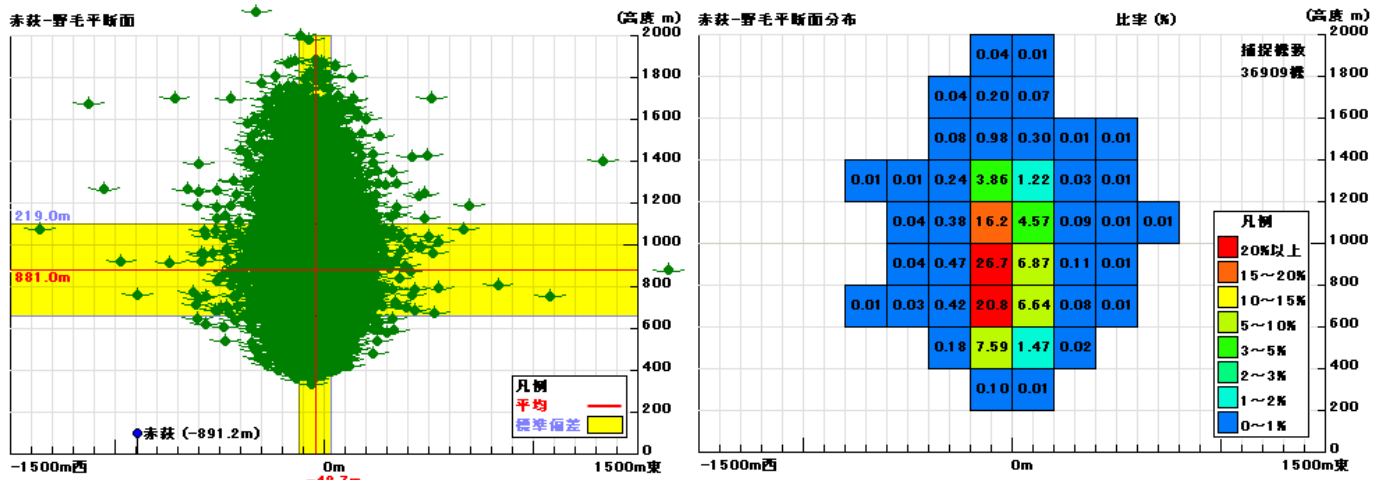
離陸機分散図
