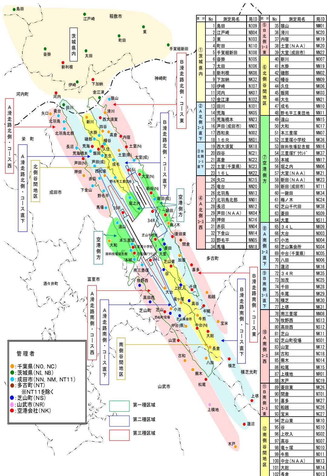
図 1-1 航空機騒音測定局配置及びエリア図
