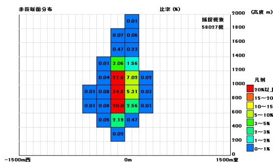
図5-2-1 A滑走路北側高度コース (赤荻断面の離陸機分布図)
