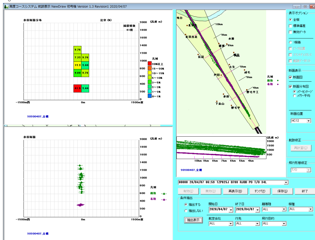
図 5-1 高度コース中央処理装置表示例
