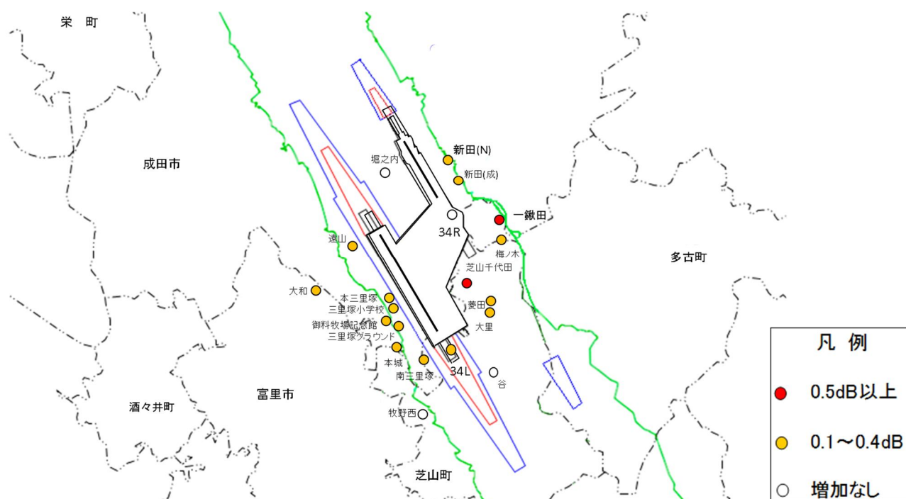
図 4-5-1 地上騒音を測定した測定局
